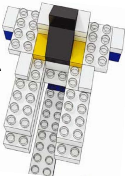
Fig. | 11 Montaje cockpit con larguero central vista superior
